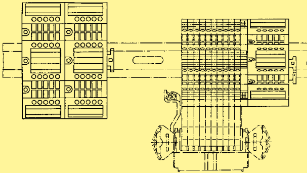
Distributor with terminal block connector Han D® AV
